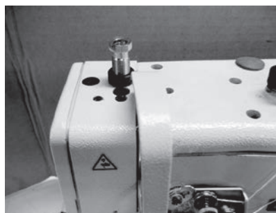
押え圧を強くしても押え棒の動きがスムーズなコイルばね仕様
