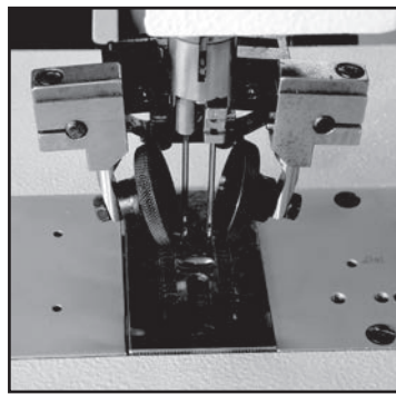
ローラー押さえ
