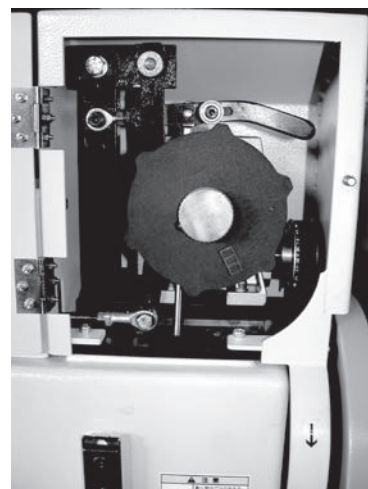
縫製パターンを変えるカム部
