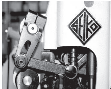
SK-2B-1-20の押え交互量調節機構
